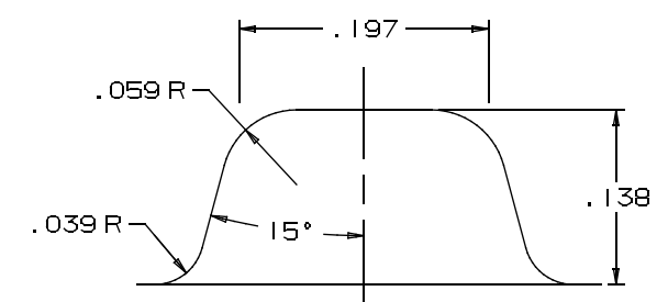
LUG DETAIL
